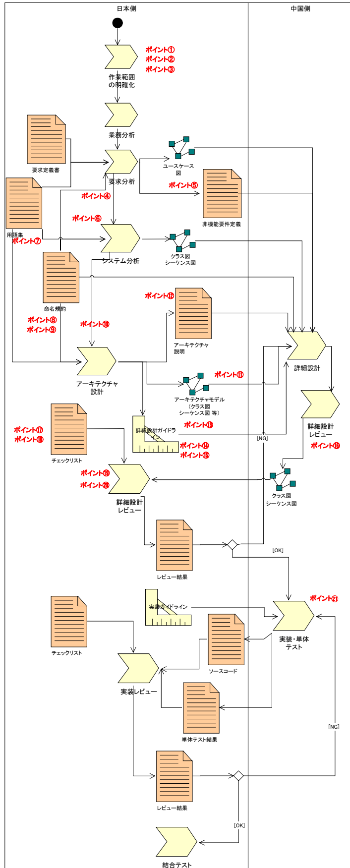
図 4.1 開発の流れ
